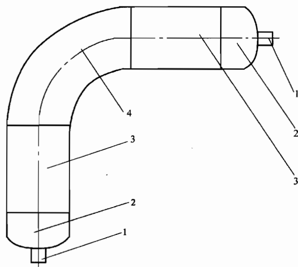
图 B-1a 弯头爆破试验试件示例
