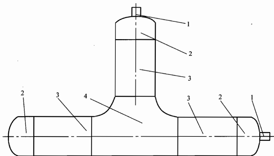
图 B-1b 三通爆破试验试件示例
