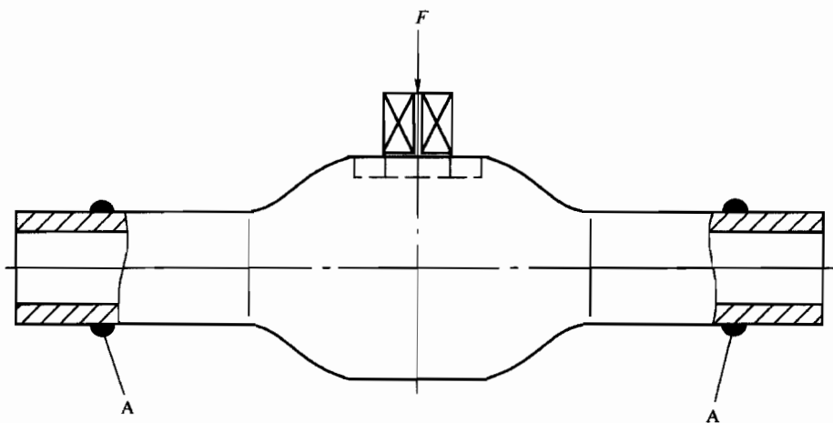
图 C-1 弯曲应力施加位置示意图
