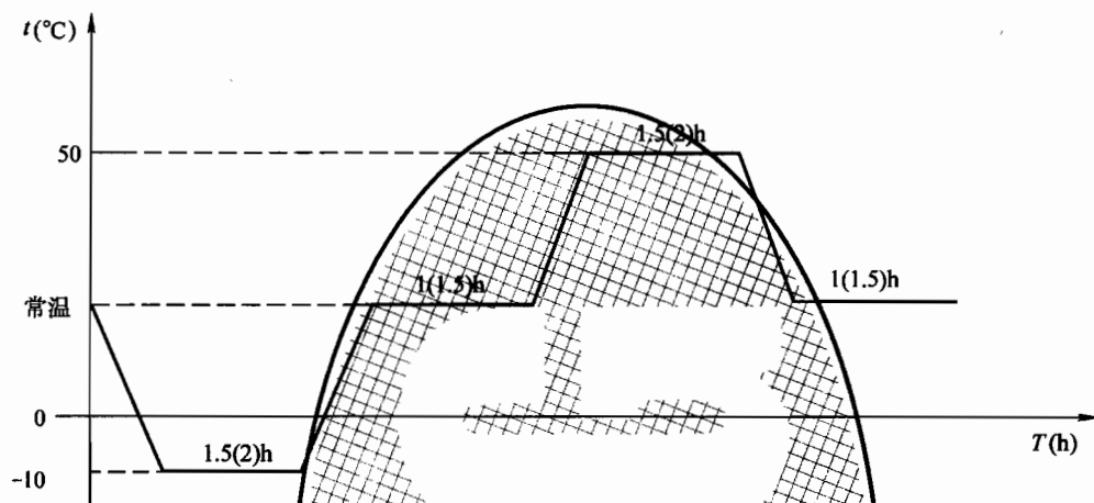
图 B-4 温度变化程序图
