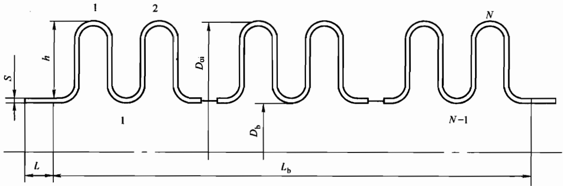
图 E-1 波纹管膨胀节疲劳试验试件尺寸图
