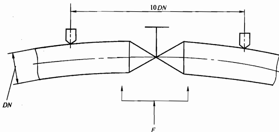
图 C-3 简支梁弯曲试验示意图( F 为施加的弯曲力)
